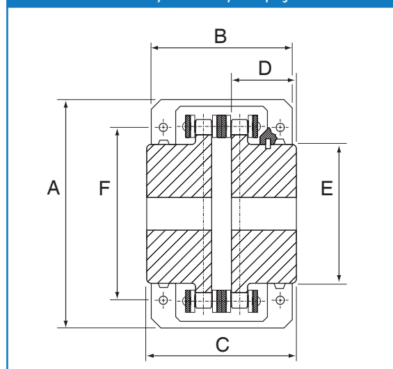
Rozměry řetězových spojek
